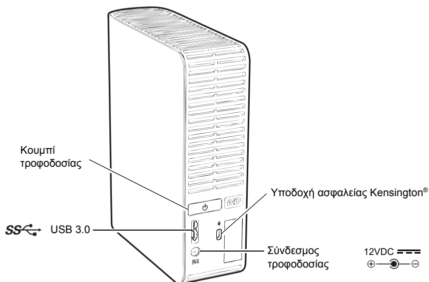
Εικόνα 3. Πίσω μέρος της μονάδας My Book Essential
